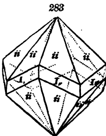
Rutile.
